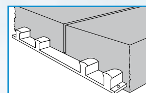
giunto esterno di ripresa di getti
