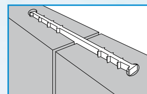
giunto interno di ripresa di getti
