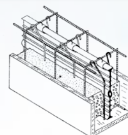
giunto esterno di ripresa di getti
