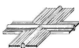
A - croce orizzontale
